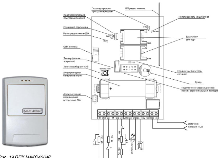
20. Плата ППК МАКС4064Р
