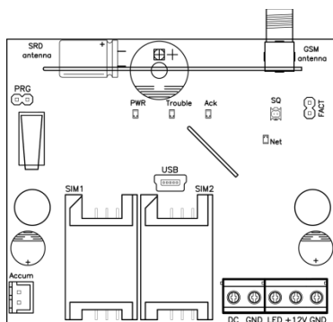
Рис. 23. Плата ППК МАКС3718Р II
