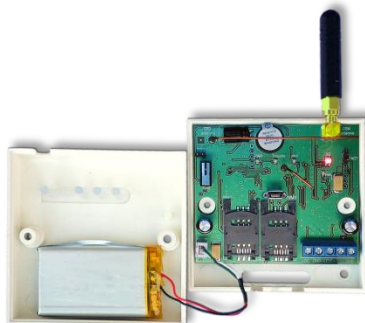
Рис. 22. ППК МАКС3718Р II с открытой крышкой корпуса
