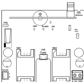
Рис. 24. Плата ППК МАКС3718Р
