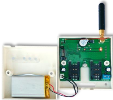
Рис. 23. ППК МАКС3718Р с открытой крышкой корпуса
