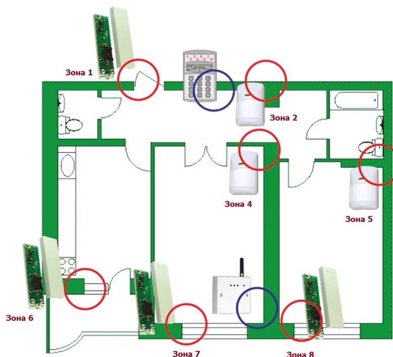
23. Размещение датчиков в квартире
