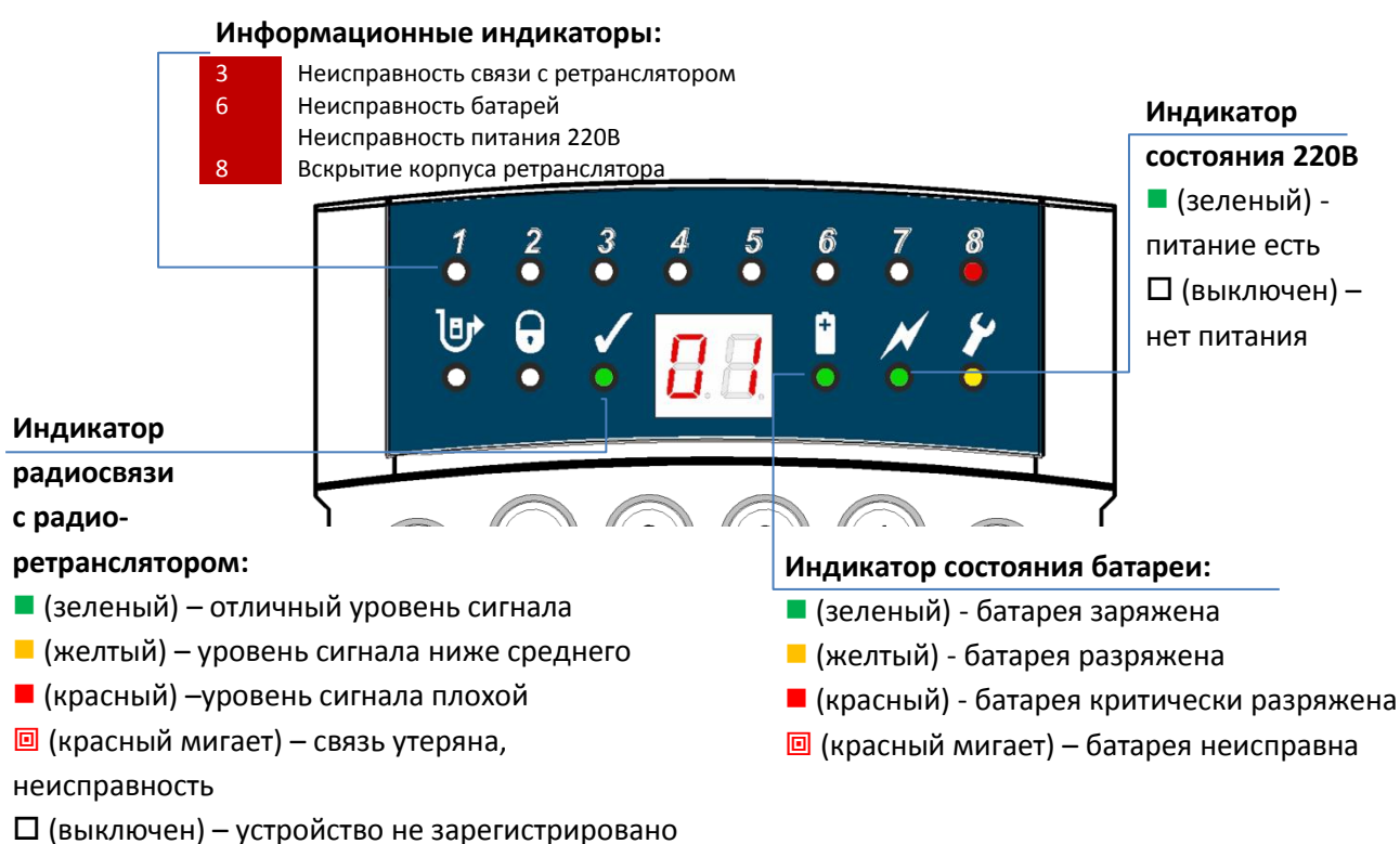
Рис. 33. Состояние радиоретранслятора
