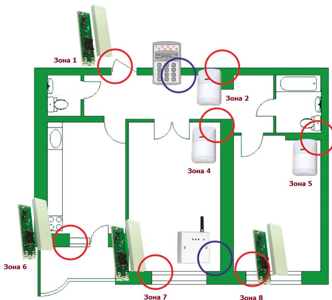
Рис. 20. Размещение датчиков в квартире
