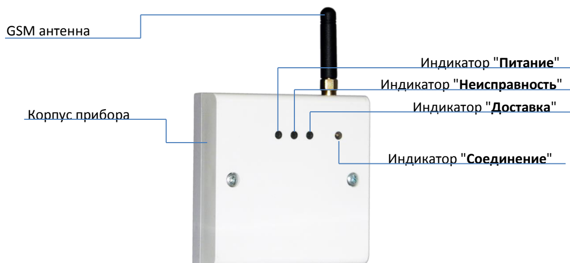
14. Прибор МАКС3718Р в корпусе
