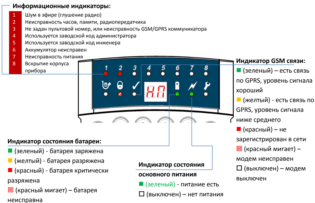
Рис. 31. Состояние прибора
