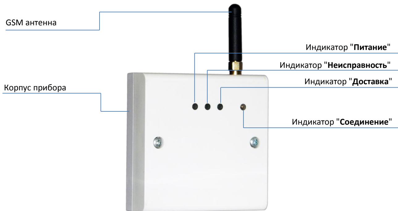
Рис. 16. Прибор МАКС3718Р в корпусе
