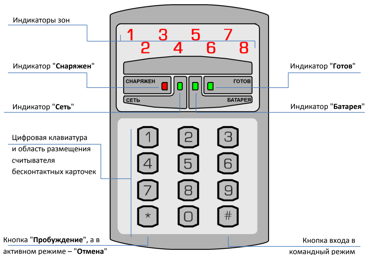
Рис. 17. Беспроводная клавиатура М8022КР
