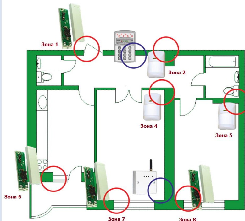
Рис. 27. Размещение датчиков в квартире
